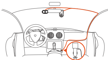
Diagrama de instalación y cableado de la lente DMS
